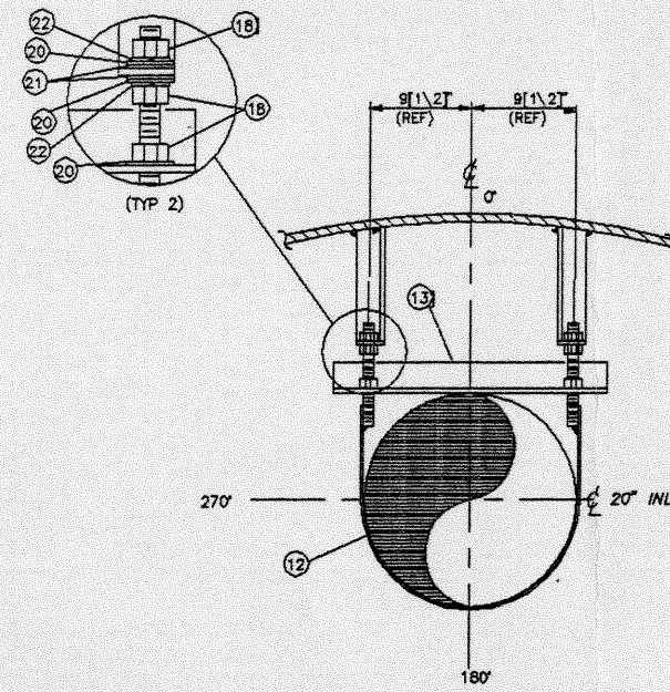
DETAIL D INLET HEADER TIE-DOWN DETAIL (TYP. 4) (N.T.S.)
